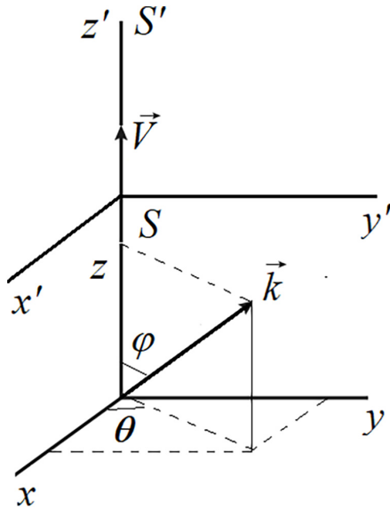
Figura 2: Onda plana eletromagnética segundo S .
