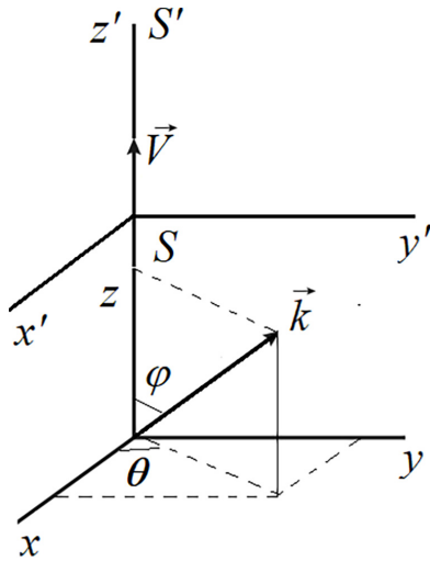
Figura 1: Sistemas de coordenadas S e S' . V é a velocidade de S' .
